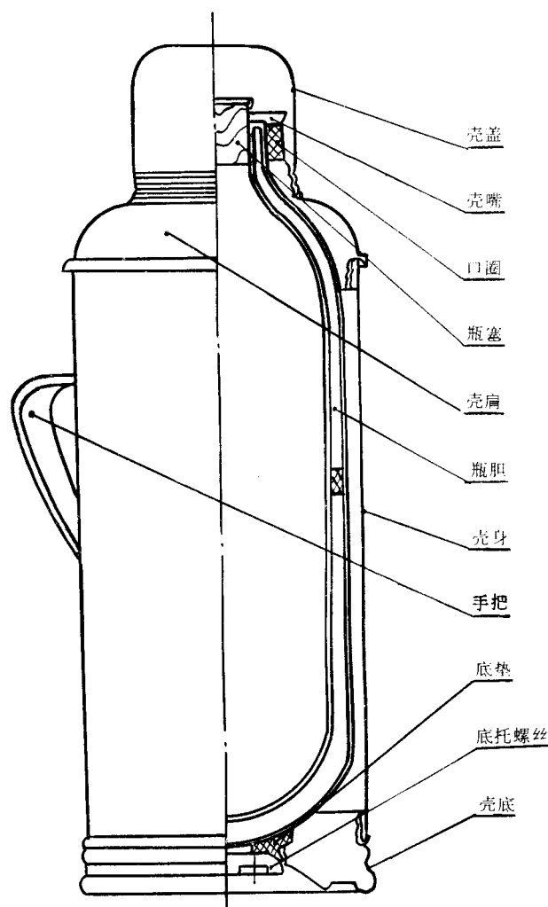
图 1 小口保温瓶结构示意图
